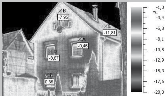
Ein Infrarotbild deckt die Schwachstellen in der Wärmedämmung auf.
